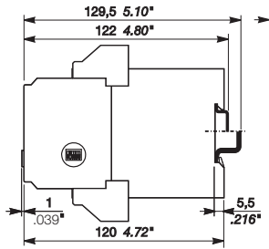
CC-U/x , CC-U/xR
