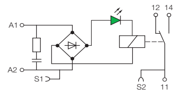
RB/RBR 121 AR
