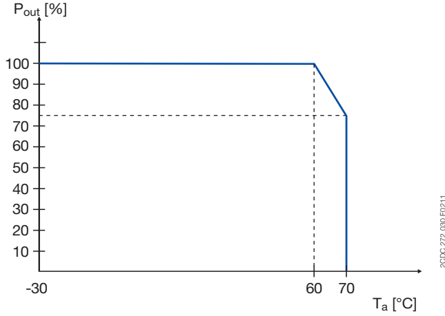
CP-T 24/20.0, CP-T 48/10.0
