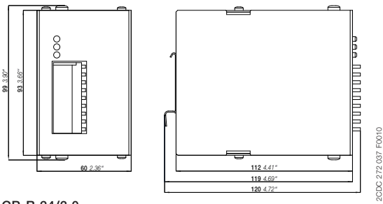
CP-B 24/3.0
