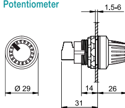
Potentiometer
