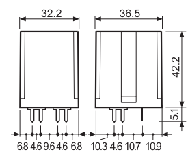
Type 65.61- 0300
