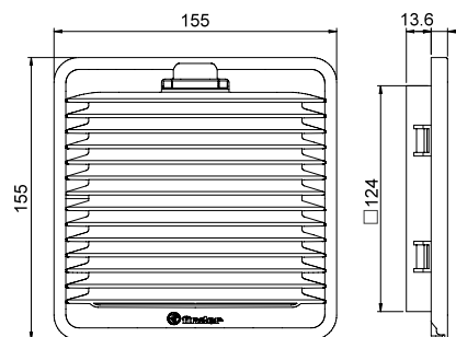
Type 7F.02.0.000.2000
