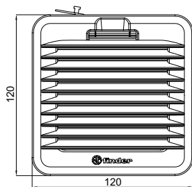
Type 7F.20.x.xxx.1020
