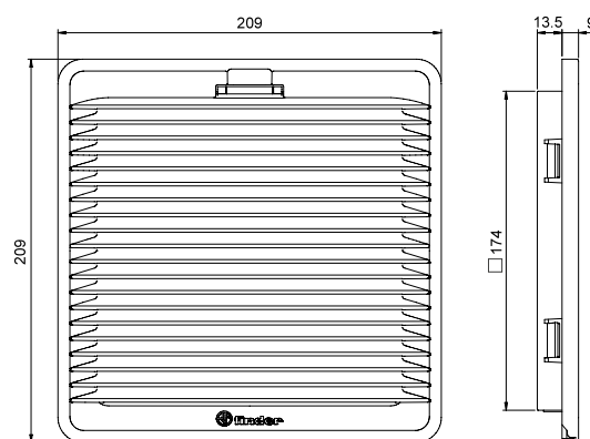
Type 7F.02.0.000.3000
