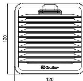
Type 7F.02.0.000.1000
